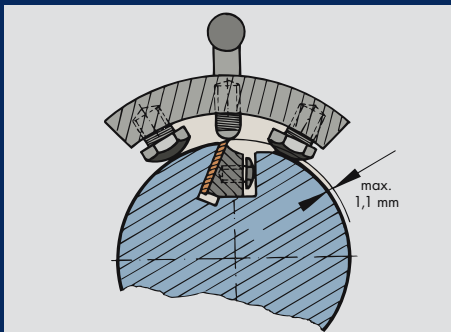
Einstellen der Hobelmesser mit Einstellehre
